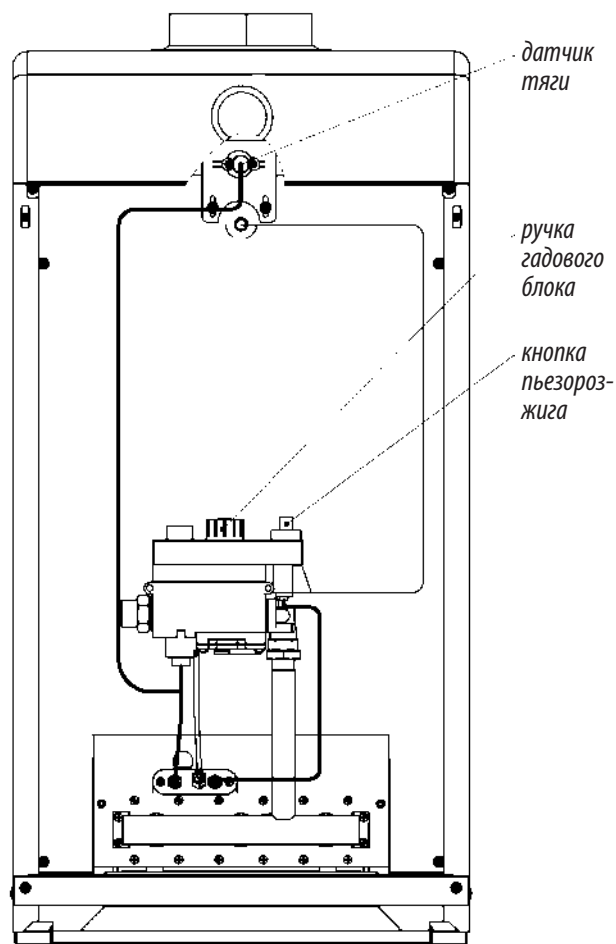
Рис.4. Особенности котлов GERKULES 20S/25S/30S с газовым блоком 710 MINISIT (дверца не показана).
