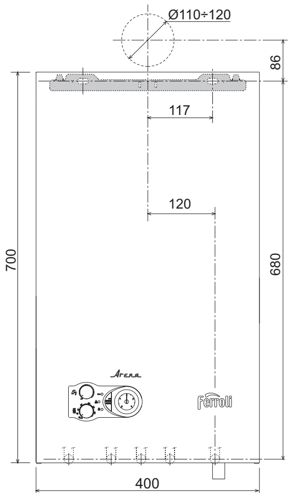
рис. 14 - Вид спереди
