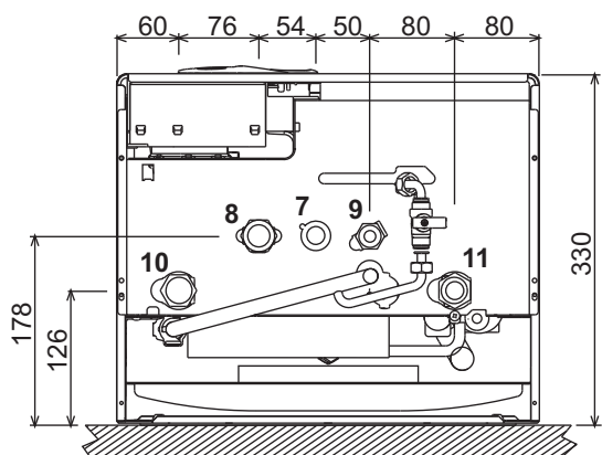
рис. 16 - Вид снизу
