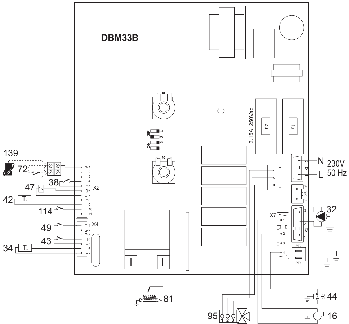
рис. 21 - Электрическая схема
