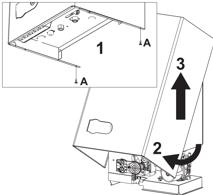
рис. 12 - Открытие кожуха
