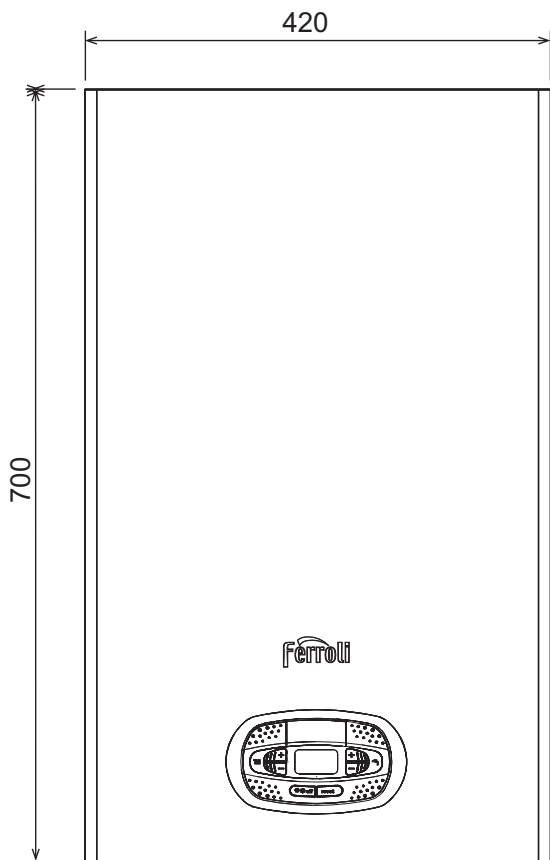
рис. 48- Вид спереди
