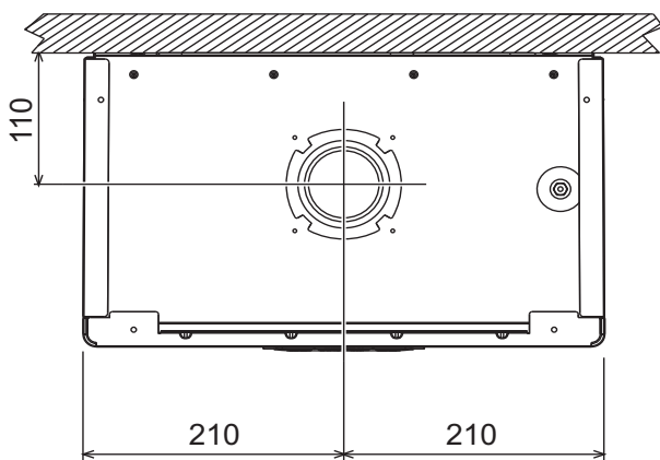
рис. 50- Вид сверху
