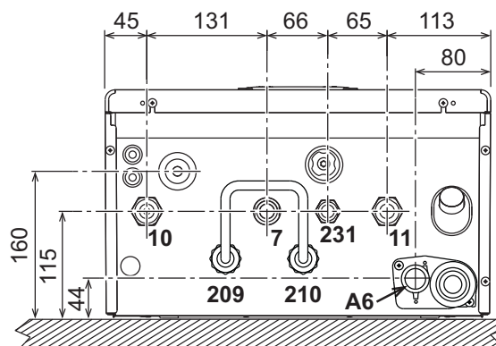
рис. 51- Вид снизу
